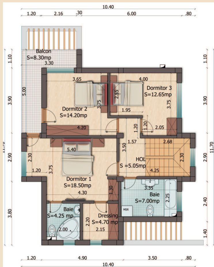
PLAN ETAJ
