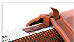
8 Element fixare coamă
