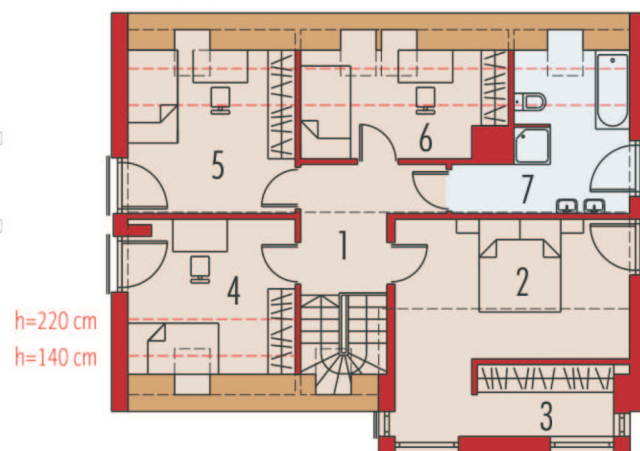
Plan ETAJ
